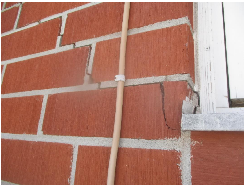
Bild 10: Spricka i tegelfasaden
