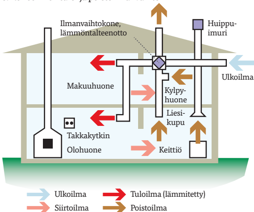
c. Koneellinen tulo- ja poistoilmanvaihto
