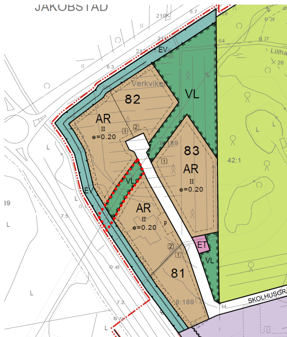
Kuva 6. Voimassa olevan asemakaavan ote. Asemakaava-alueen ohjeelliset rajat on merkitty punaisella katkoviivalla.
